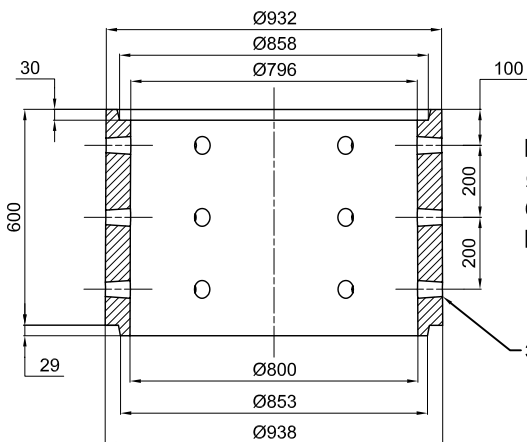
BUSE DE PUIITS A EMBOITEMENTS Ø Int. 0,80 m Ht. 0,60 m - PERFOREE
